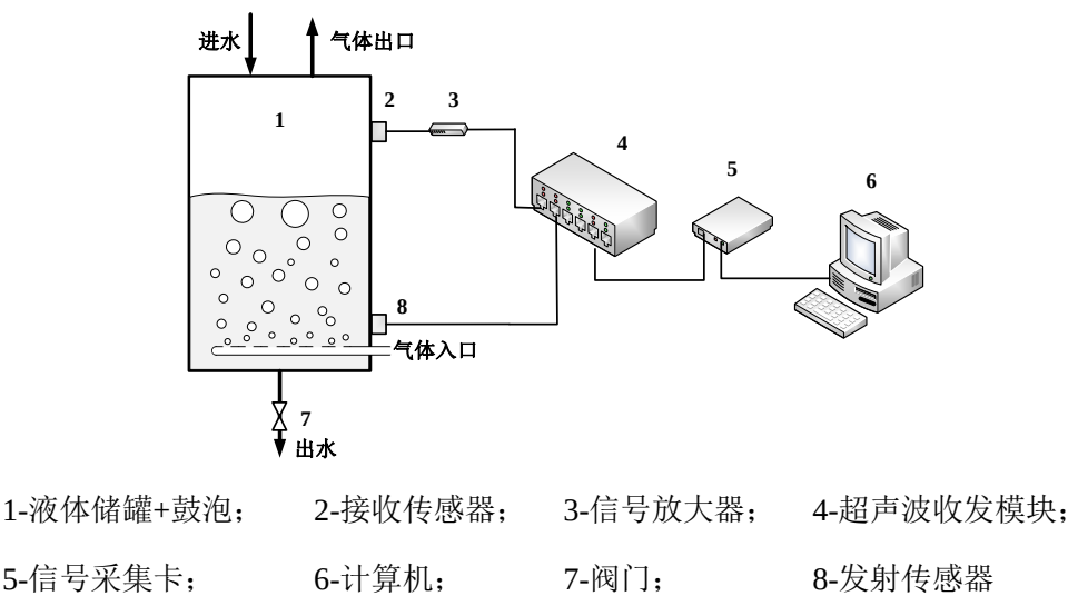
图 8 超声波液位检测示意图
