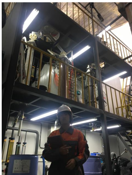
(c) 制备清洁柴油的加氢反应冷模装置 (氢气鼓泡进入柴油)
