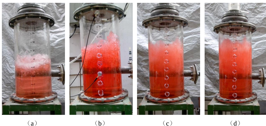
图 10 鼓泡塔“拟稳态”液位测量实物图
