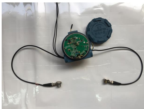
图 23 超声波液位检测仪样机实物照片
