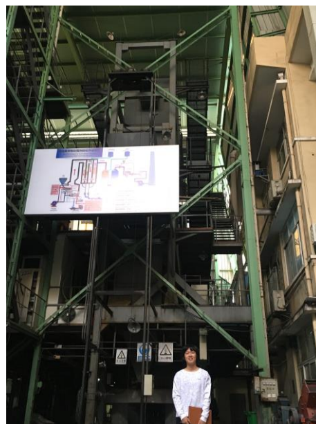
(d) 制备醋酸的射流反应器 (液体向下射流, 气体向上鼓泡)
