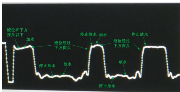
图 13 鼓泡装置动态液位测量时接收信号幅值随时间的变化（截屏图）
