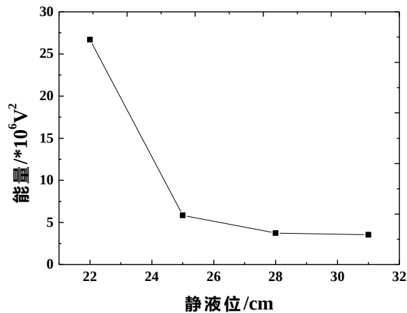
图 11 接收到的声信号能量与静液位之间的关系
