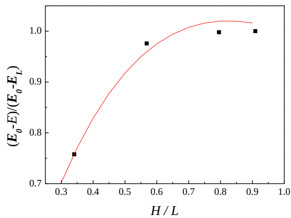
图 12 鼓泡装置无因次声能量随无因次液位高度的变化
