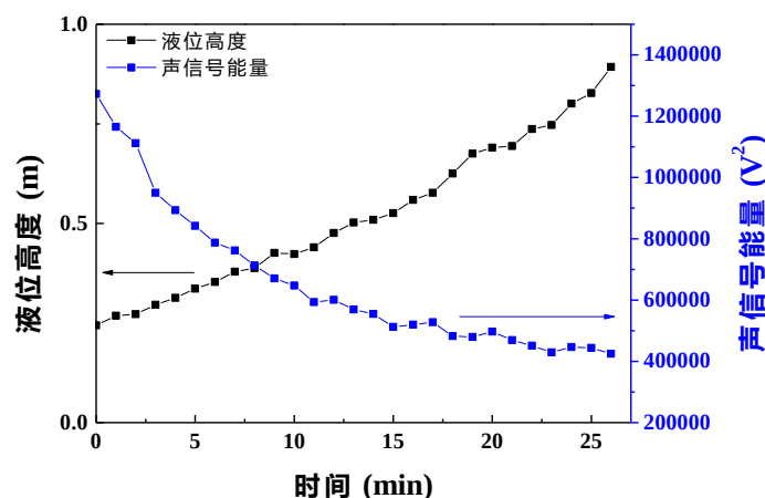
图 16 活鱼运输箱液位高度与超声波能量之间的关系
