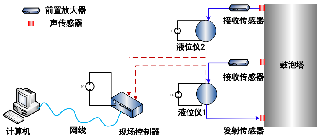
图 24 鼓泡塔超声波液位检测示意图
