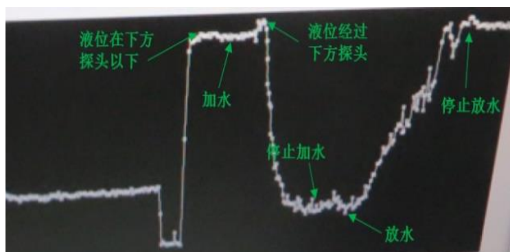
图 14 鼓泡装置中鼓泡区液位测量时接收信号幅值随时间的变化（截屏图）
