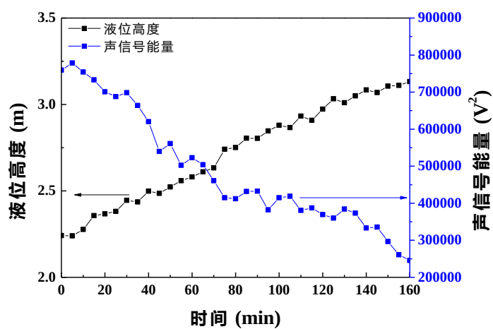
图 19 液位高度与超声波能量之间的关系
