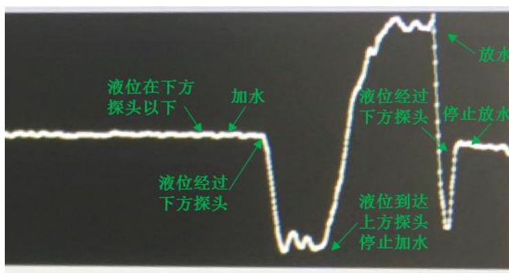
图 9 动态液位（加水、放水过程）测量时接收信号幅值随时间的变化（截屏图）
