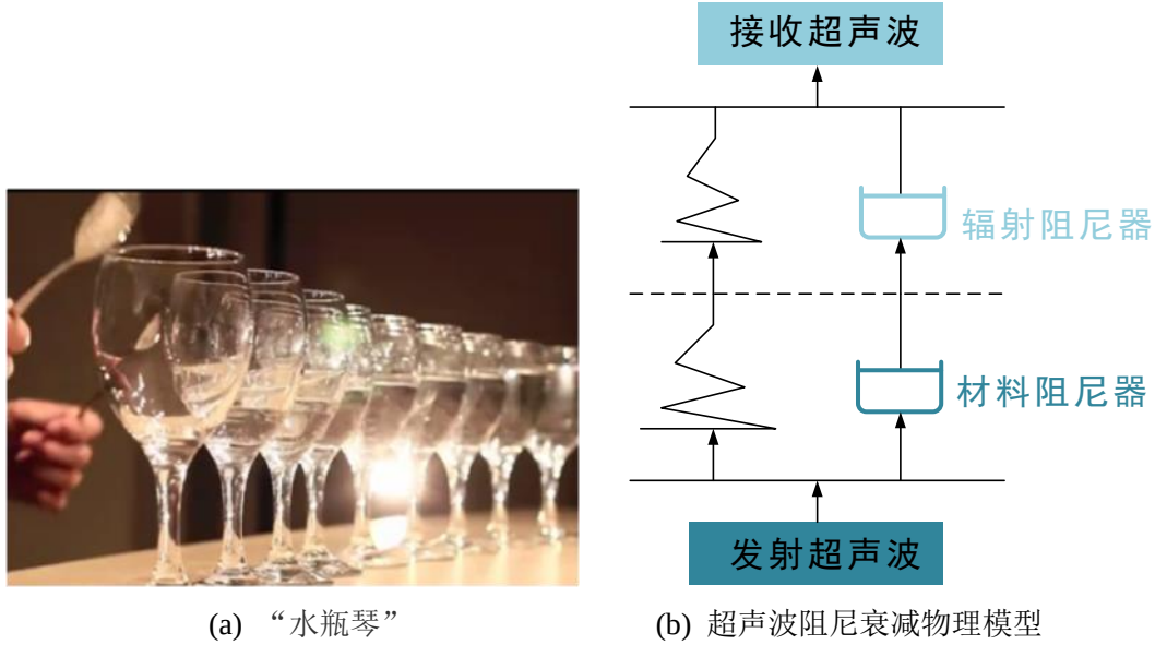
图 6 基于超声波阻尼衰减的液位检测原理
